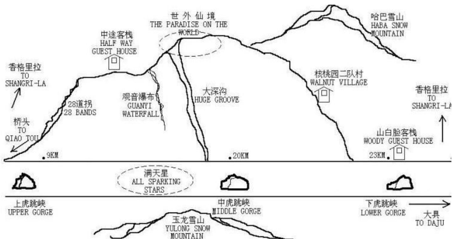
虎跳峡景区示意图
