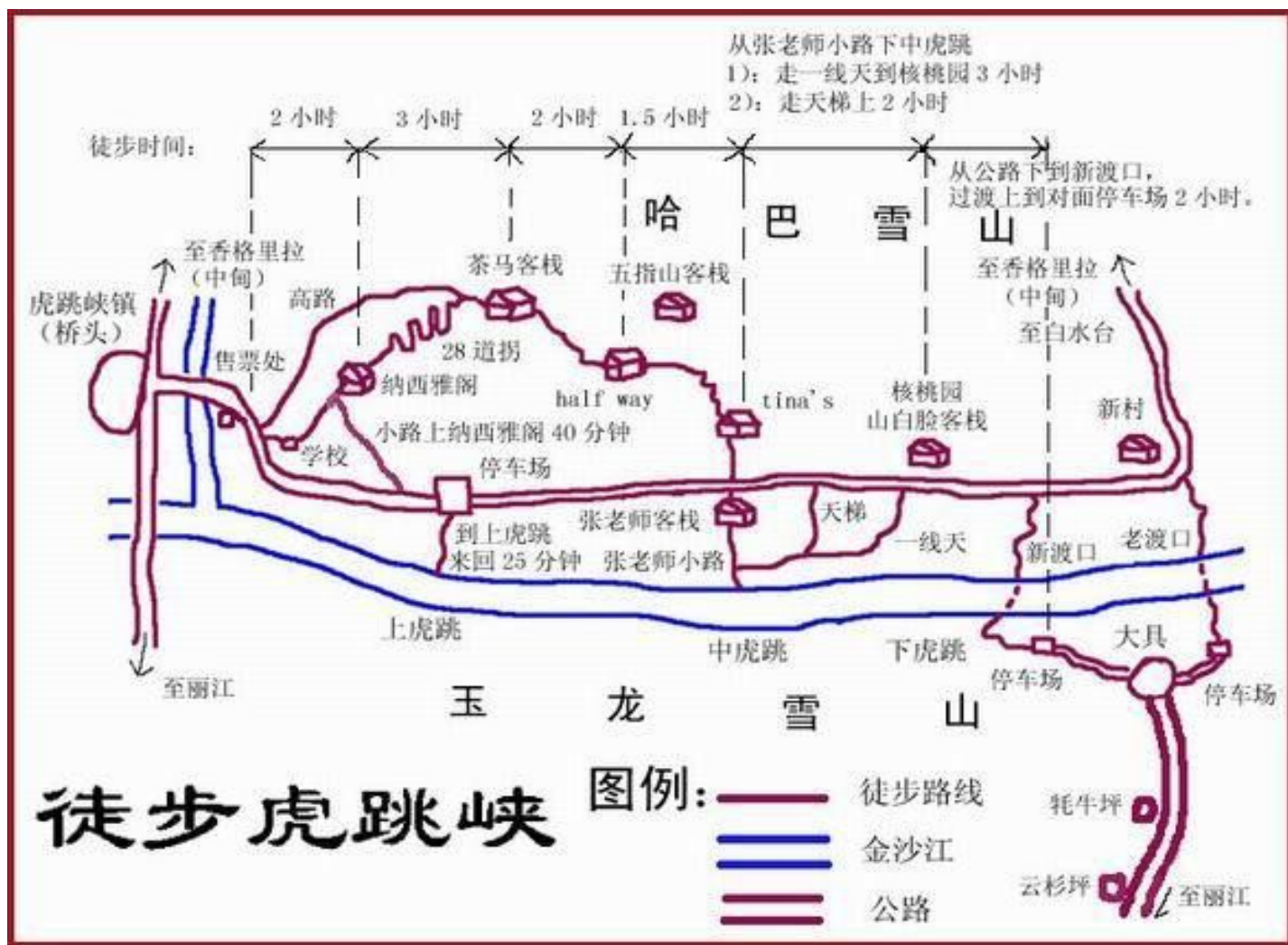
虎跳峡徒步路线
